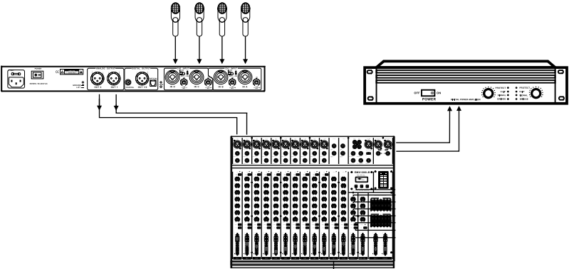
图5 插入话筒通道
