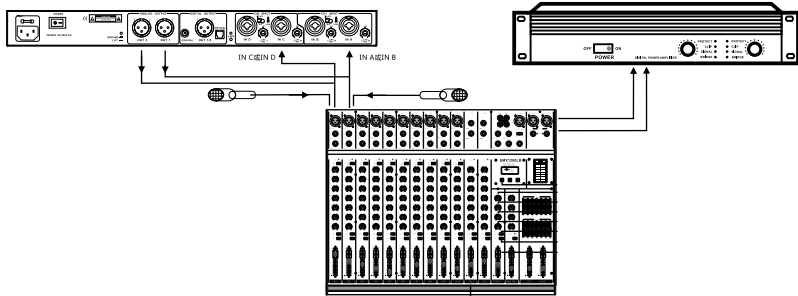
图1 插入话筒通道
